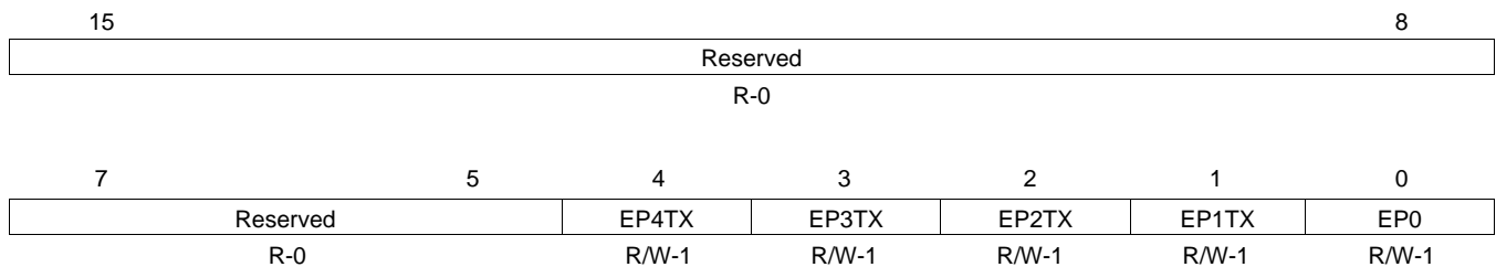
Figure 64. Interrupt Enable Register for INTRTX (INTRTXE)
